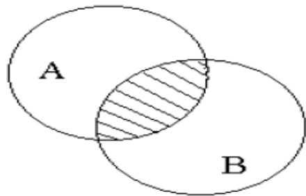
Рис.2 Пересечение множеств
