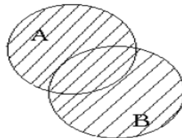
Рис.3 Объединение множеств
